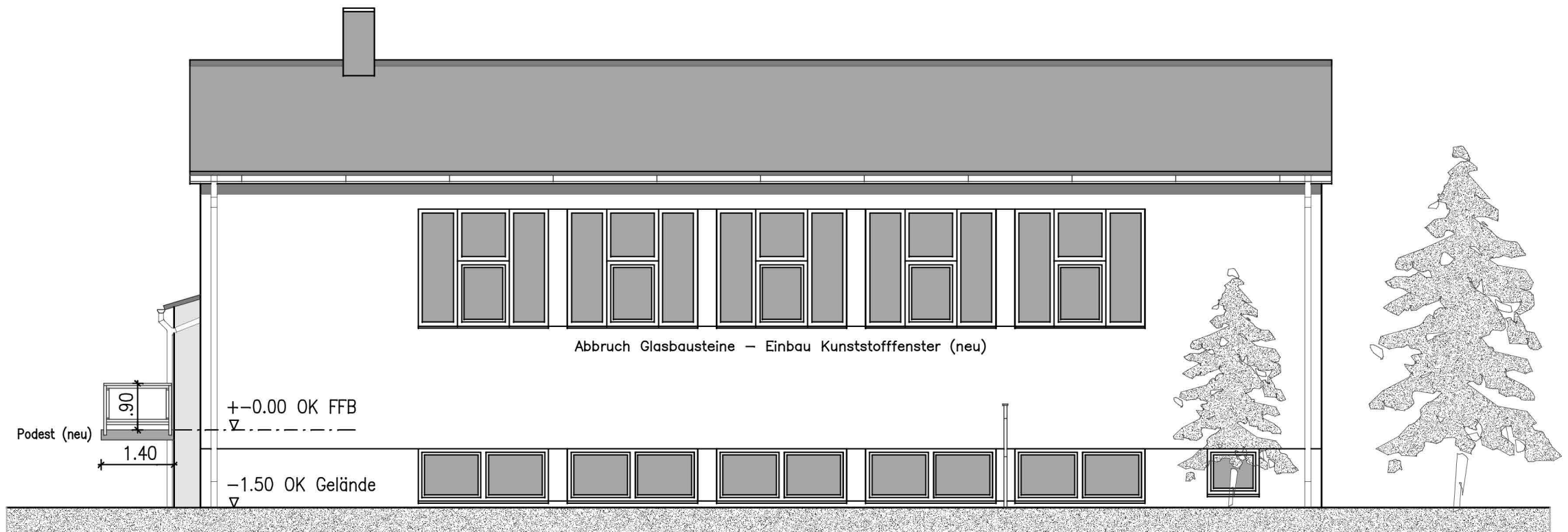
WESTANSICHT
